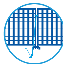
Installation de la jambe de force avec un crayon
